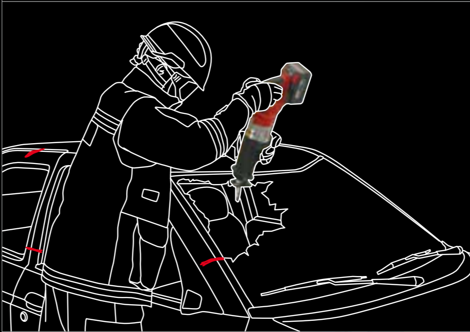
2 Glas zwischen Schnittpunkten entfernen Remove glass between the cutting points
