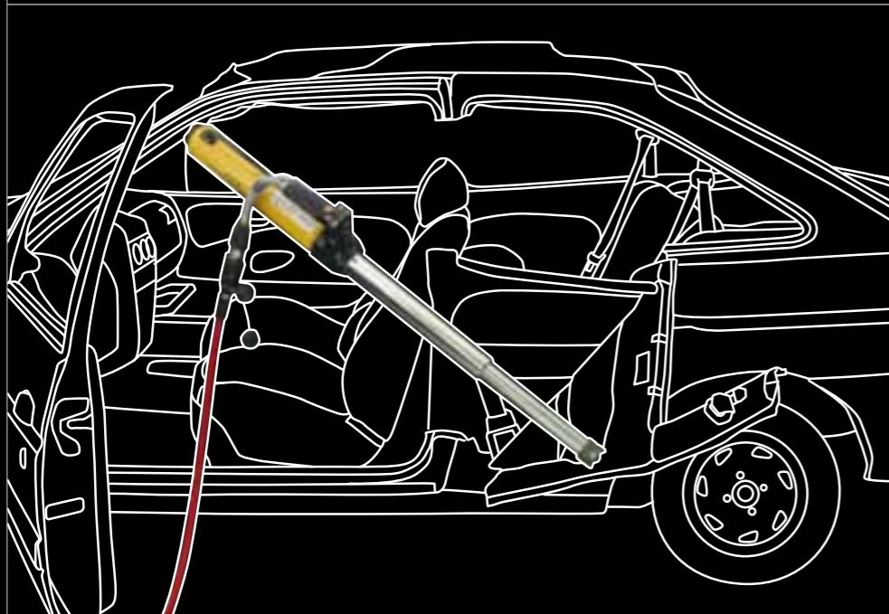
3 Rettungszylinder ausfahren Extend rescue ram
