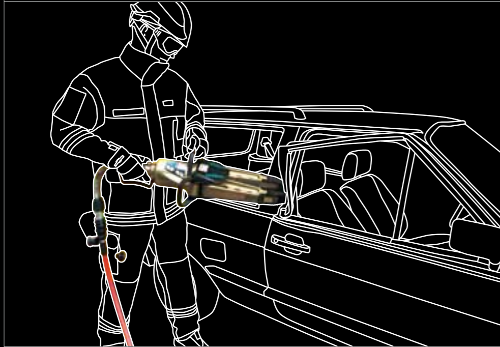
1 Fensterrahmen wegbiegen Bend window frame open
